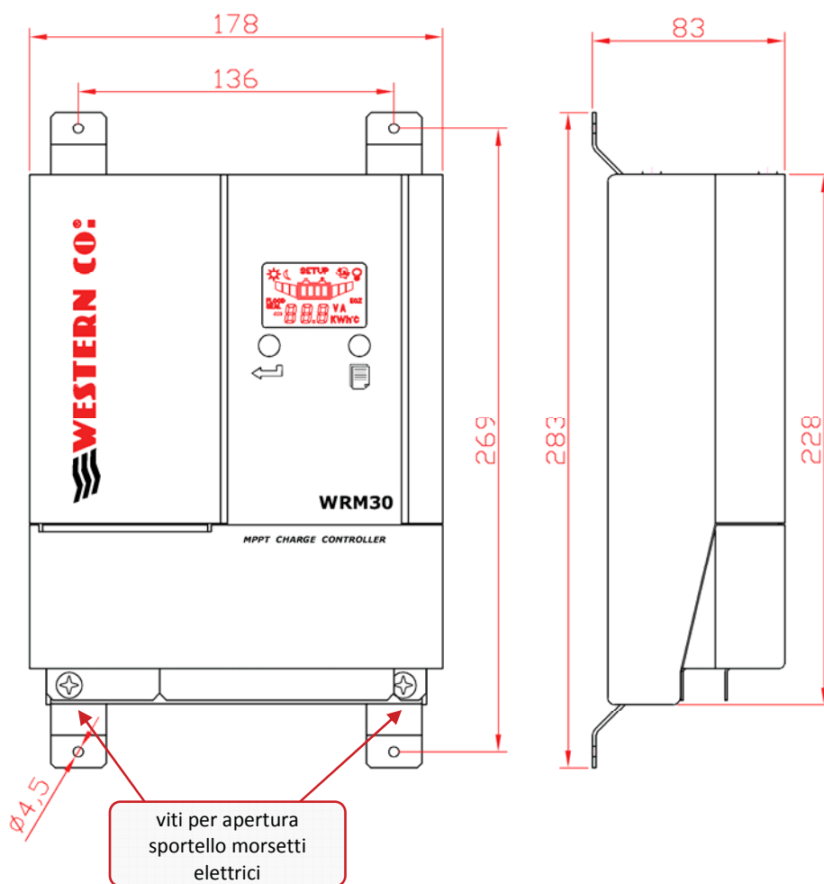
Fig. 4 Dimensioni (mm)
