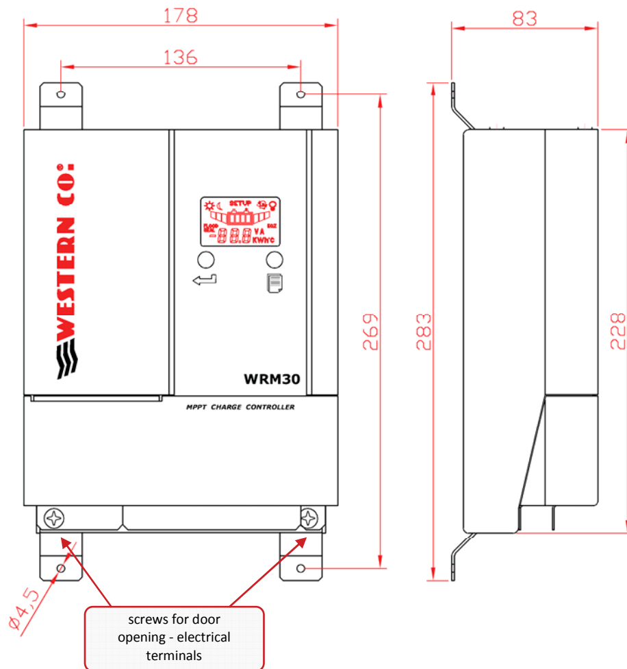
Fig. 4 Dimensions (mm)
